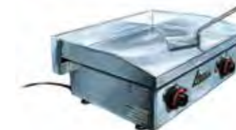
785 Placa de snack plancha 220 V / 16A monofásica - 3,3 kW. Ext. : L 60 l 40 Alt. 19 cm. Temperatura maxi 300°C. Se sirve con cajón para grasa. 59 Kg
